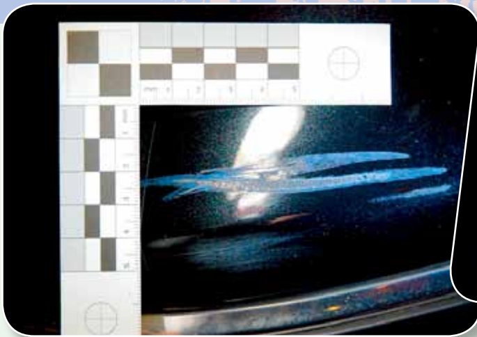
▲圖12、直接使用閃光燈垂直照射物面所產生明顯的光斑。
