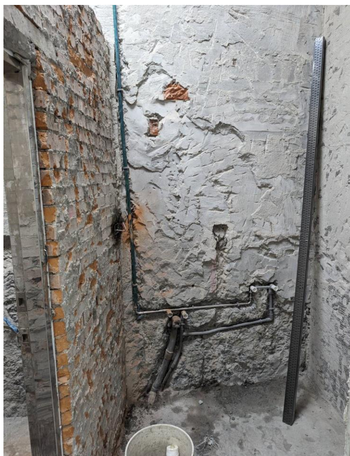
6（女警待勤室浴廁施工中）
