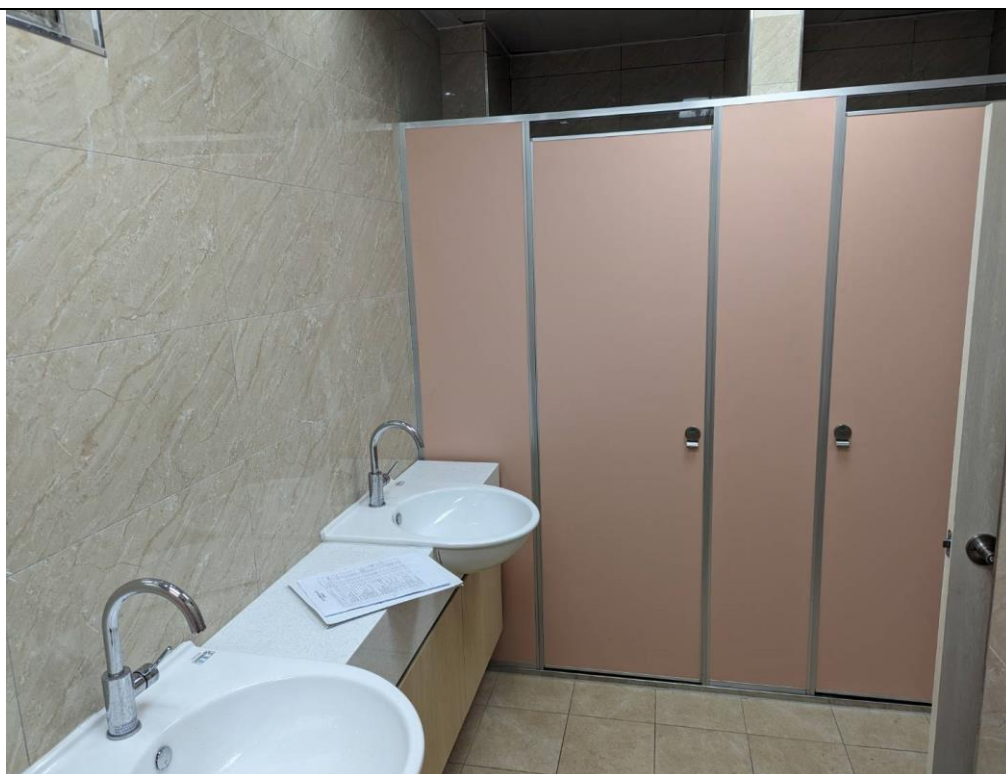
13 (3樓待勤室浴廁施工後)
